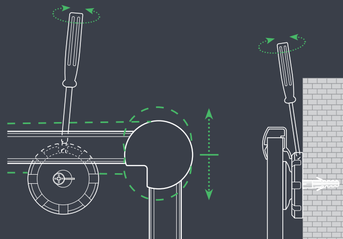
Leichte Montage: Bequem das Board MAULpro nach dem Aufhängen bis zu 6 mm nachjustieren mit patentiertem MAUL-Exzenter-Element
