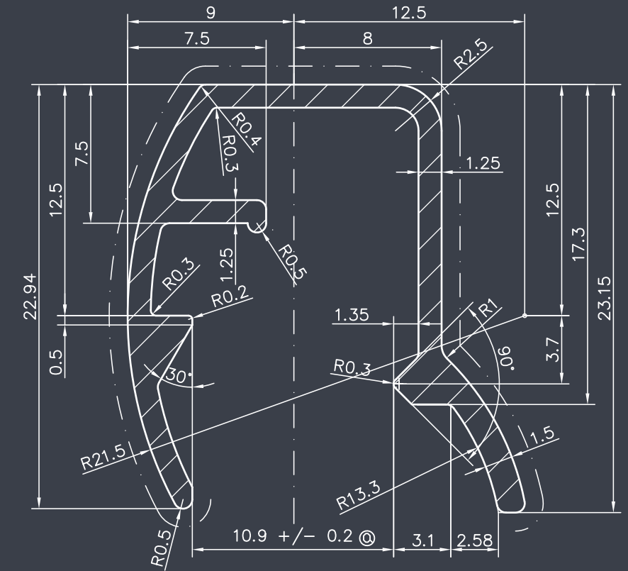
Präzision bis ins Detail: Querschnitt des Aluminiumprofils für das Whiteboard MAULpro
